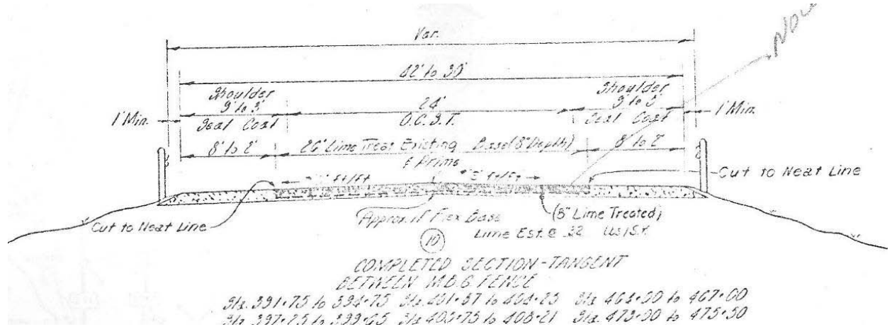
b) SH 49 Pavement
