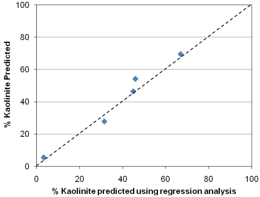
a) Kaolinite Mineral
