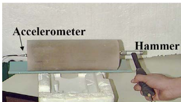
a) FFRC Test Setup
